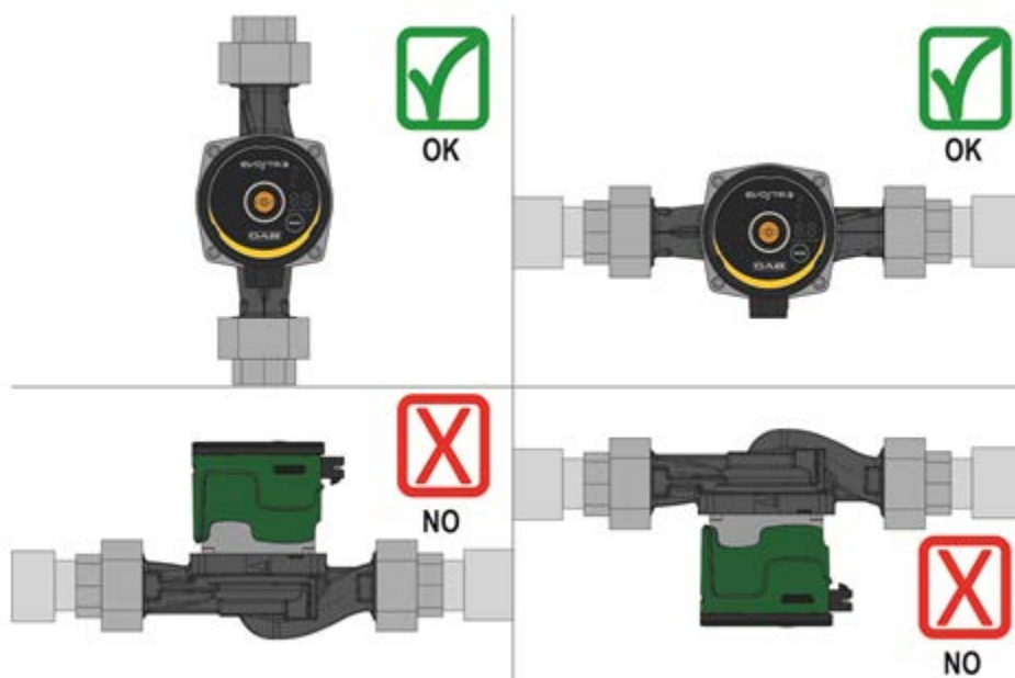
Obrázek.3: Poloha montáže
